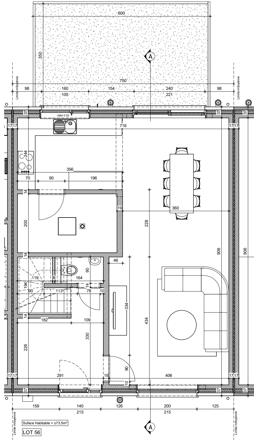
REZ-DE-CHAUSSEE
